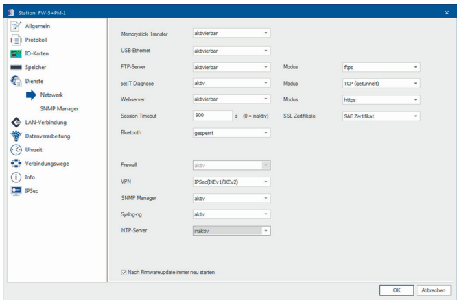
Auswahl der Dienste und Funktionen in setIT
