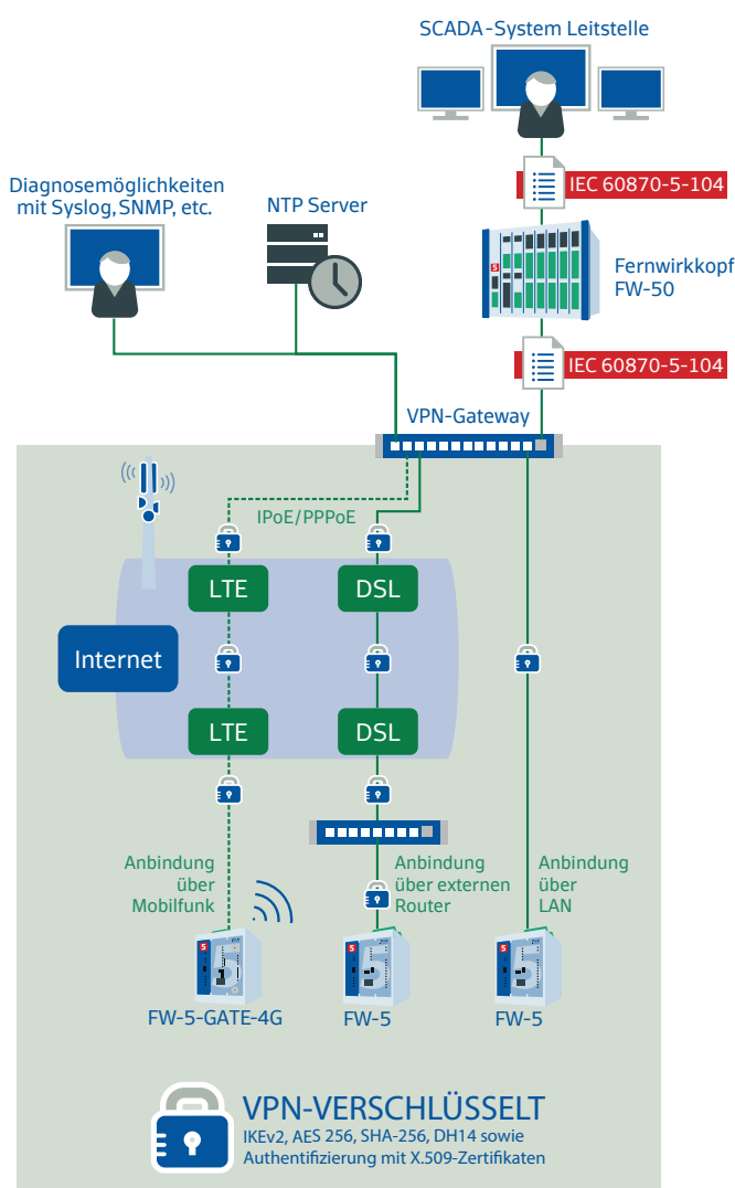
Anbindungskonzept - Flexible und sichere Einbindung von Fernwirktechnik
