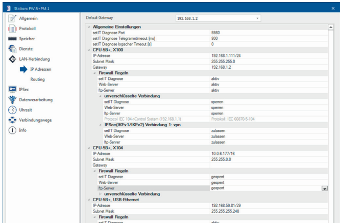
Firewall mit Verbindungseinstellungen über VPN in setIT
